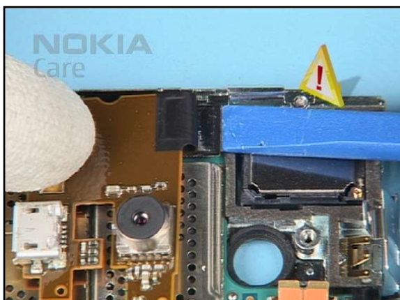
23. Open the AV FLEX connector and remove the AV FLEX ASSEMBLY.
